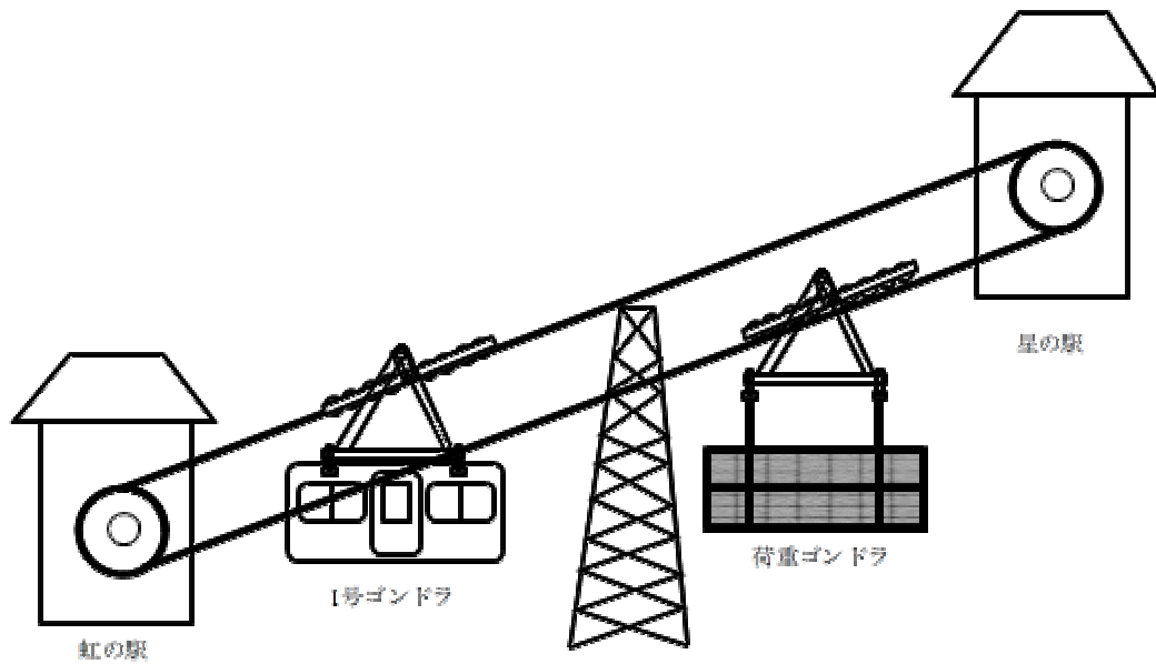
片線運行のイメージ図
